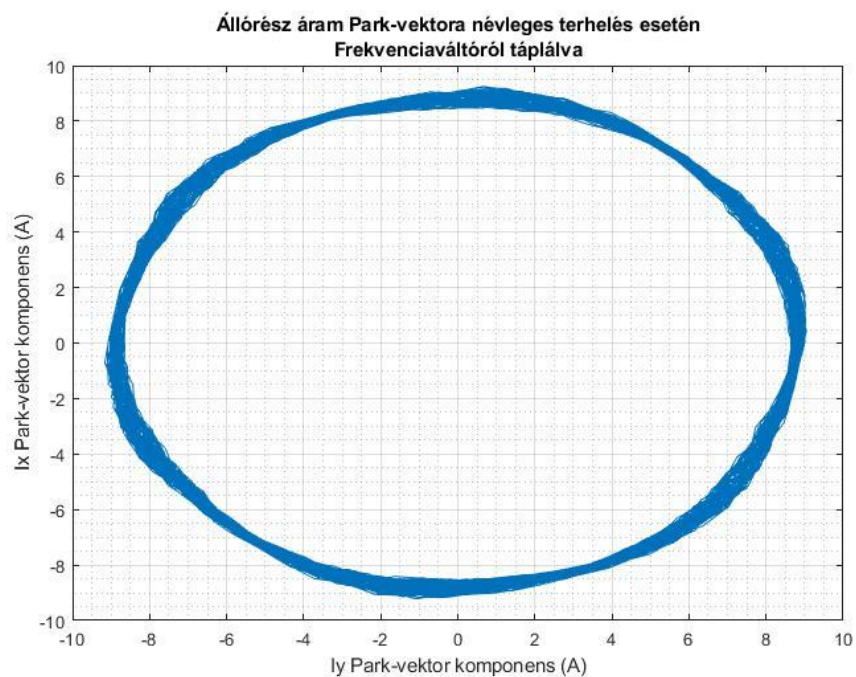
4.2. ábra Háromfázisú aszinkronmotor állórész áram Park-vektor jellege terhelte üzemállapotban.
