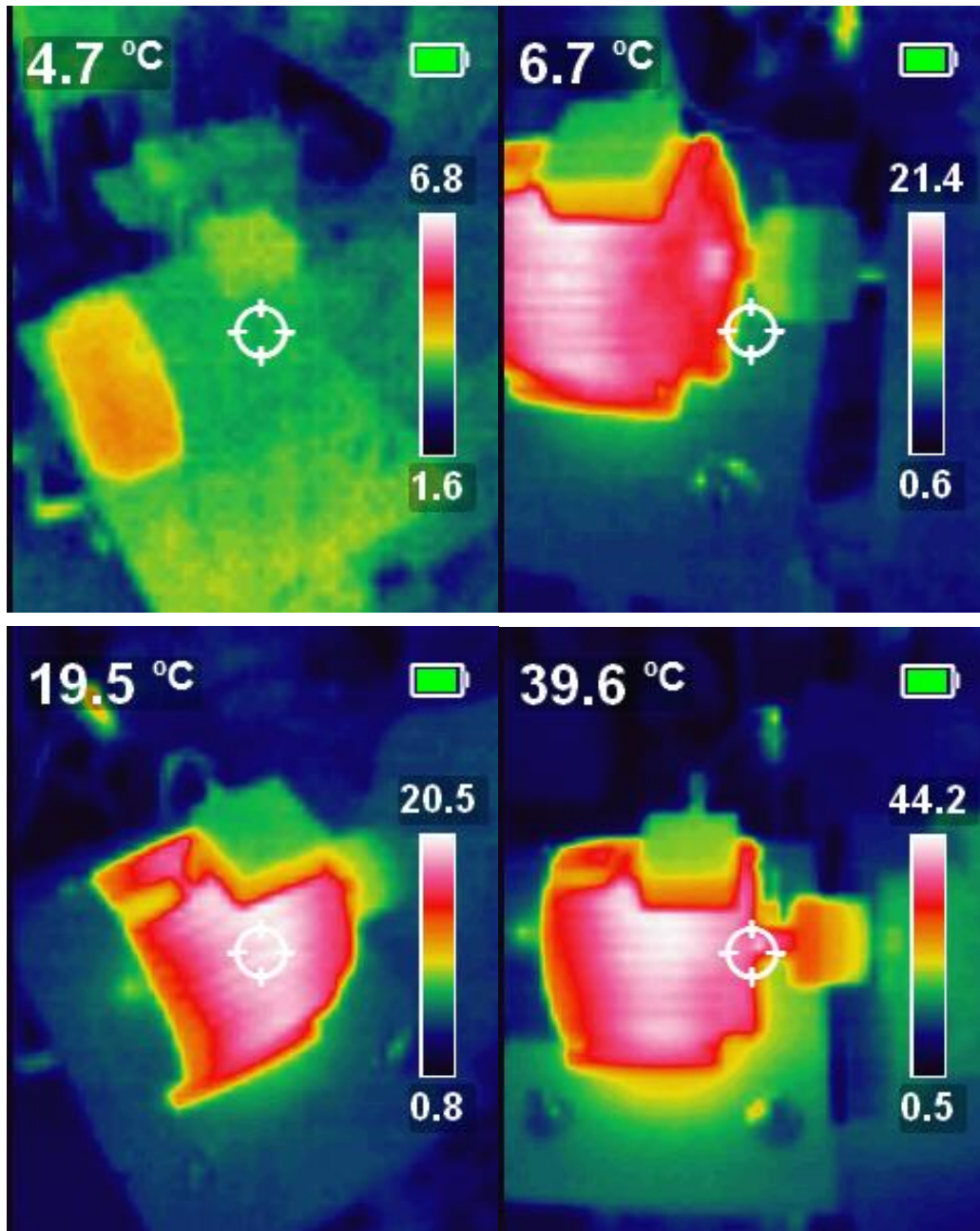
2.9. ábra. Aszinkron motor tengelykapcsolójának és motorház felületének aszimmetrikus melegedése.
