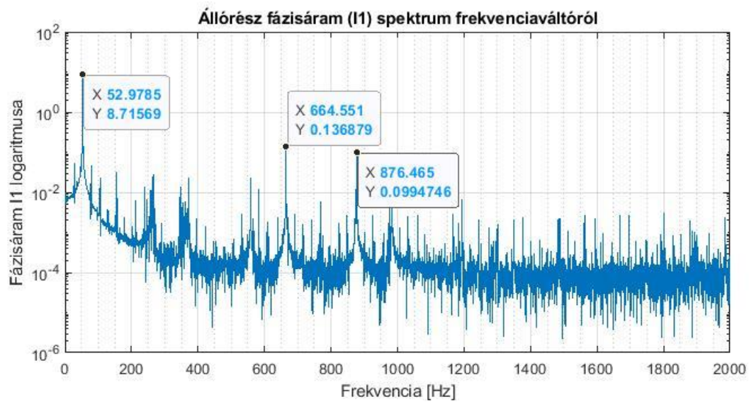
4.3. ábra. Állórész áram I_1 fázisáram spektrumának képzése frekvenciaváltós üzemben, FFT.
