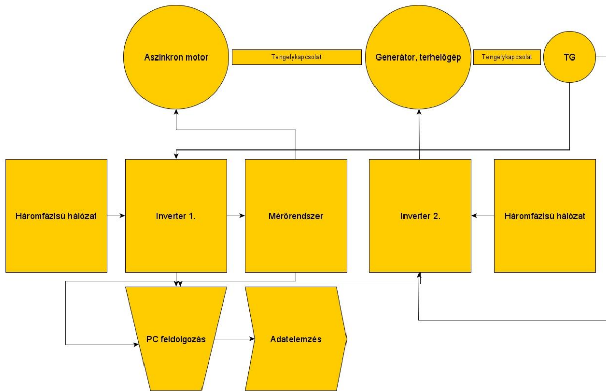
2.5. ábra Egyszerűsített mérési elrendezés blokkvázlata [25].
