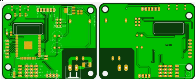
Sl. 2. Izgled štampane ploče senzorskog čvora
